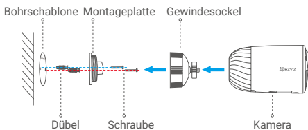
Abb. 2 Montage auf Gewindegewinde
