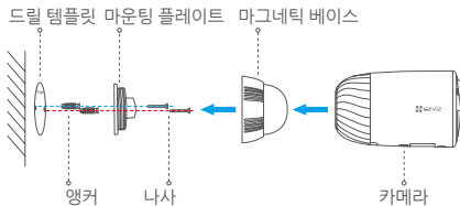
그림 1 마그네틱 베이스로 장착
