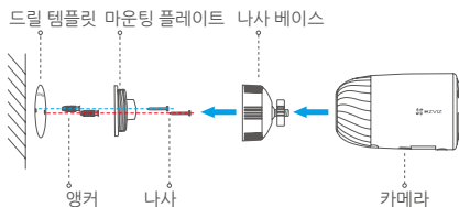
그림 2 나사 베이스로 장착
