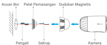
Gambar 1 Pemasangan dengan Dudukan Magnetis
