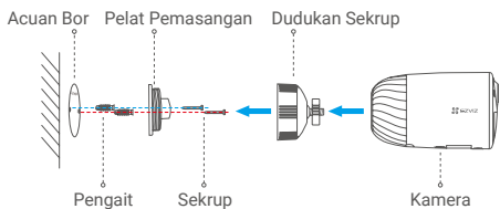
Gambar 2 Pemasangan dengan Dudukan Sekrup
