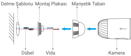
Şek.1 Manyetik Tabanla Monte Etme
