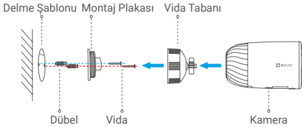
Şek.2 Vida Tabanı ile Monte Etme
