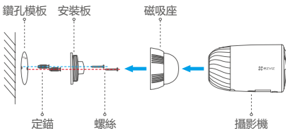
圖 1 使用磁吸座安裝
