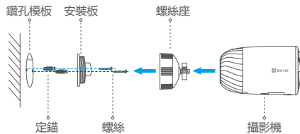
圖 2 使用螺絲座安裝
