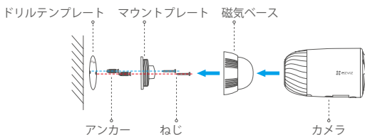
図1 マグネットベースによる取り付け
