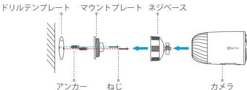
図2 ネジベースによる取り付け
