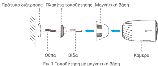
Εικ.1 Τοποθέτηση με μαγνητική βάση
