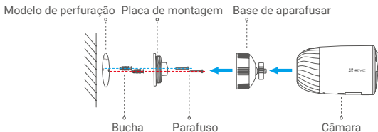
Fig.2 Montagem com base aparafusada
