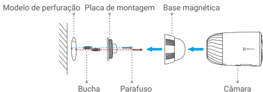
Fig.1 Montagem com base magnética
