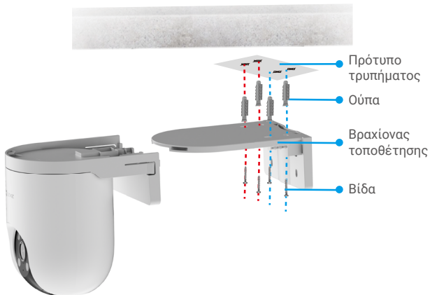
Εικ. 1 Τοποθέτηση στην οροφή
