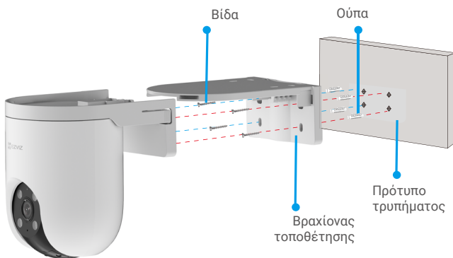
Εικ. 2 Τοποθέτηση στον τοίχο
