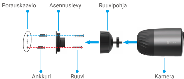
Kuva 2 Asennus ruuvipohjalla
