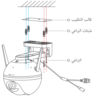
الشكل 2 التركيب في السقف
