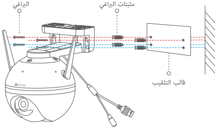
الشكل 1 التركيب على الجدار
