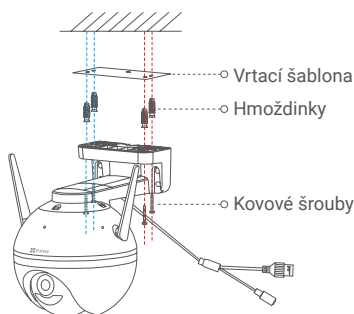
Obr. 2 Stropní montáž
