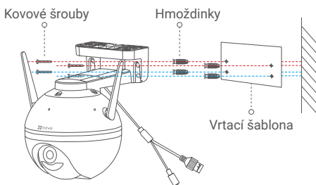
Obr. 1 Nástěnná montáž
