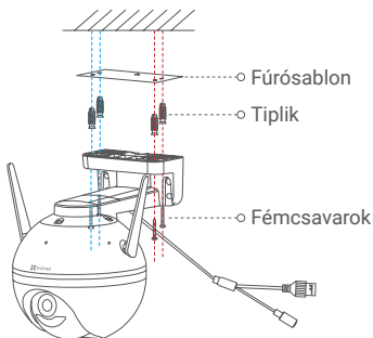
2. ábra Szerelés mennyezetre
