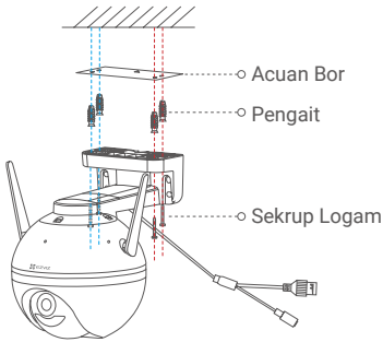
Gambar 2 Pemasangan pada Plafon
