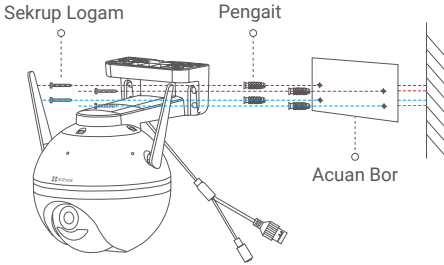
Gambar 1 Pemasangan pada Dinding
