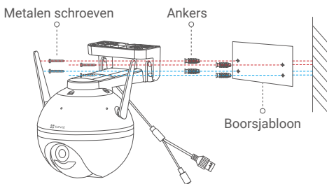
Afb.1 Muurmontage
