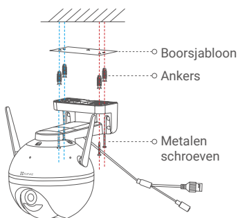
Afb.2 Plafondmontage
