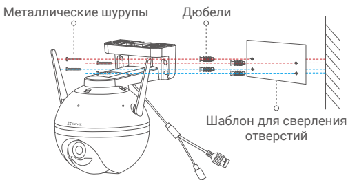
Рисунок 1. Настенный монтаж
