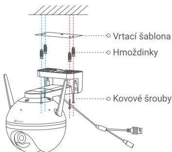
Obr. 2 Stropní montáž
