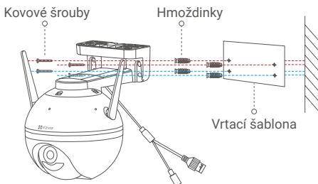
Obr. 1 Nástěnná montáž
