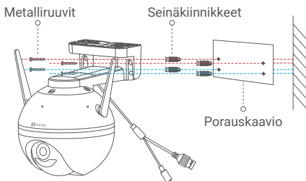
Kuva 1 Seinäasennus
