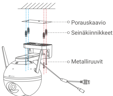
Kuva 2 Kattoasennus
