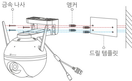
그림1 벽면 설치
