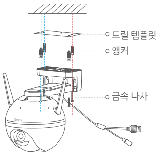
그림2 천장 설치
