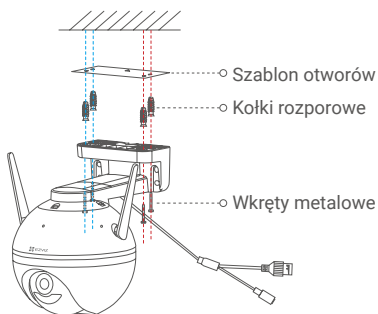
Rys. 2 Montaż sufitowy
