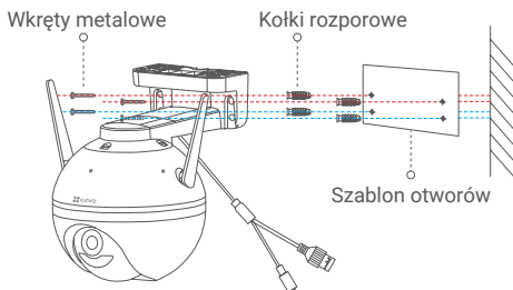
Rys. 1 Montaż ścienny
