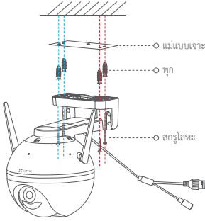
รูปที่ 2 การติดตั้งบนเพดาน
