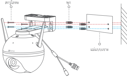
รูปที่ 1 การติดตั้งบนผนัง
