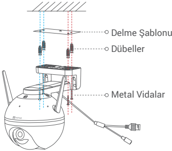
Şek.2 Tavana Montaj
