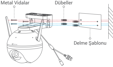
Şek.1 Duvara Montaj
