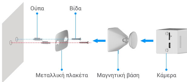
Εικ. 2 Στερέωση με βίδες
