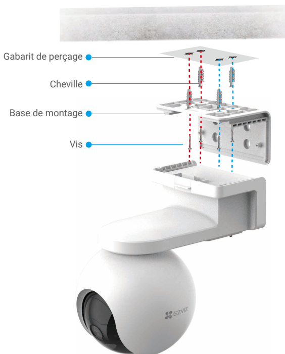
Fig. 1 Montage au plafond
