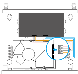
Stromanschluss
