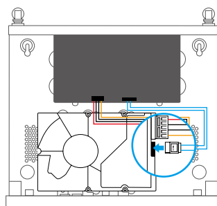
Dátové rozhranie
