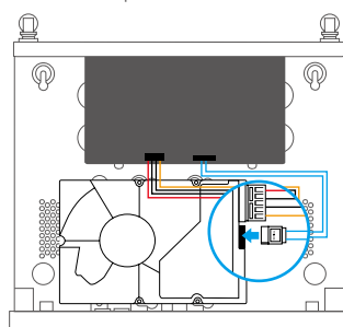
Datenanschluss
