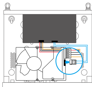
Dataport
