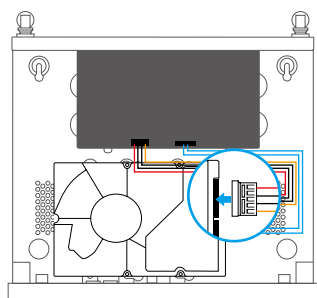
Rozhranie napájania
