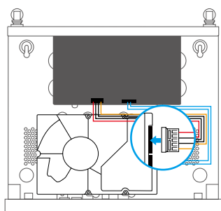
Interface d'alimentation
